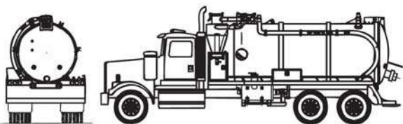
DOT407, TC407, DOT412, TC412 Tanque cargado al vacío (TC350)
