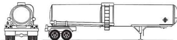
DOT407, TC407, SCT 307 Autotanque de baja presión para productos químicos (MC307, TC307)
