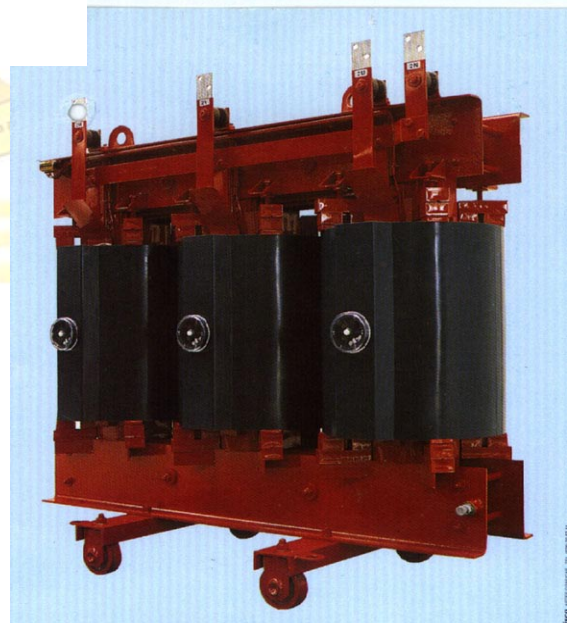
Fig. 13: Transformador seco.
