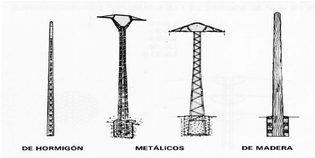
Fig. 5: Tipos de apoyos.
