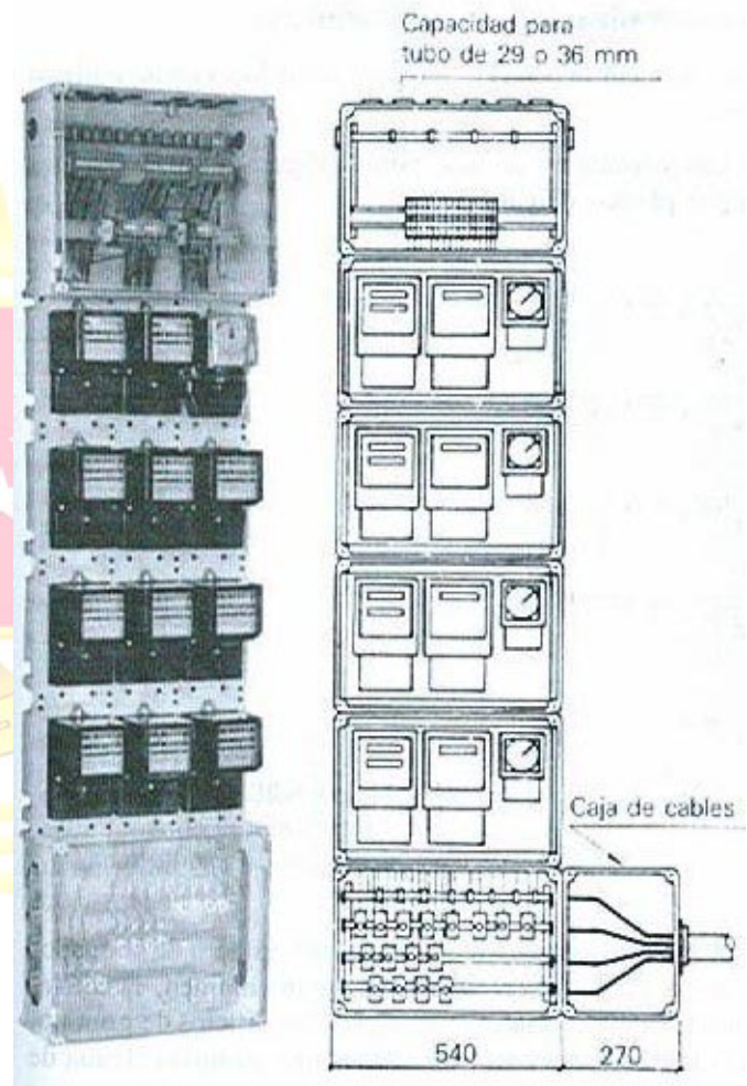
Figura: Centralización de contadores. Embarrado en la parte inferior, contadores en el medio, y módulo de salida en la parte superior.
