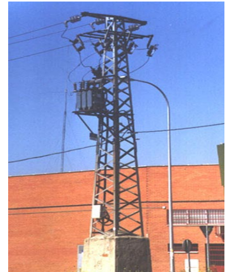
Fig. 9: Transformador de intemperie o aéreo
