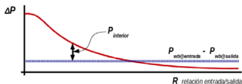
Imagen 151. Saldo de presión interior en una técnica de VPP en contra del viento.
