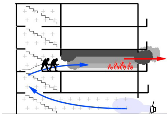
Imagen 127. Comparativa del desplazamiento de los gases de incendio en el acceso a una vivienda en altura desde la caja de escaleras con la misma sin presurizar o presurizada.
