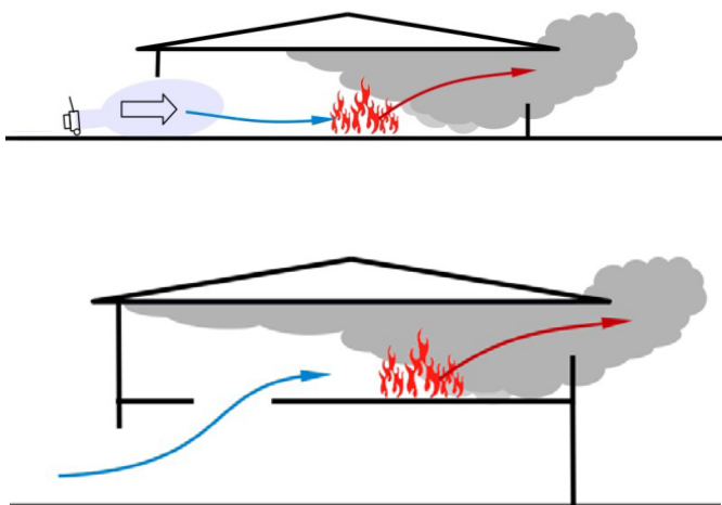
Imagen 171: Ejemplos de flujo de gases que generan bien una entrada o una salida de gases a través de las aperturas. Son flujos unidireccionales.
