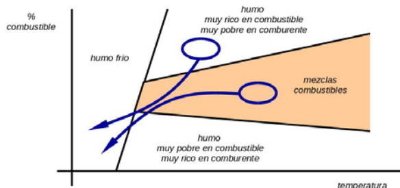
Imagen 43. Efecto de enfriamiento y dilución mediante aplicación de agua.
