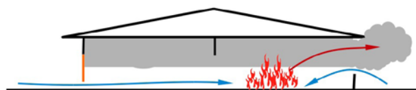
Imagen 111. La colocación de una cortina de bloqueo de humo (en naranja) permite transformar el flujo bidireccional en la entrada en un flujo unidireccional que facilita el acceso de bomberos.
