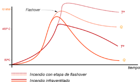
Imagen 26. Evolución comparada de la temperatura (T) y potencia (Q) en un incendio infraventilado frente a un incendio que transcorre por una etapa de flashover .
