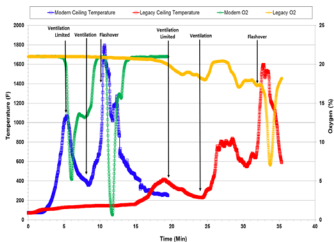
Imagen 34. Evolución de la temperatura y las concentraciones de oxígeno en el experimento de Underwriters Laboratories comparando la evolución de un incendio con combustible moderno y otro con tradicional en una misma vivienda reproducida a escala real.
