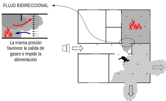
Imagen 121. Ventilación VPP defensiva sin el confinamiento del recinto de incendio. El flujo bidireccional se mantiene tras el inicio de la ventilación. Tan pronto sea posible deberá confinarse el incendio.
