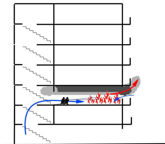
Imagen 181: Ataque interior con ventilación natural
