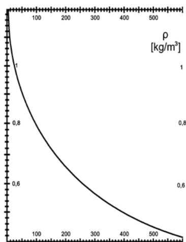
Imagen 12. Gráfica variación de la densidad del aire en relación con la temperatura
