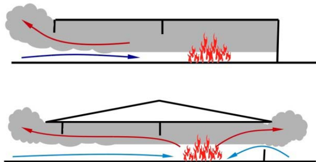
Imagen 172: Ejemplo de flujo bidireccional en las aperturas.
