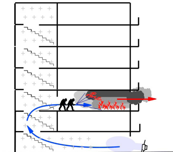
Imagen 182: Ataque en presión positiva para la extinción.
