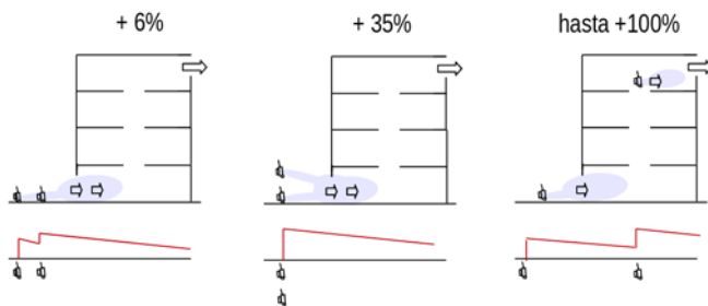
Imagen 147. Comparación del aumento del caudal efectivo con distintas combinaciones de ventiladores
