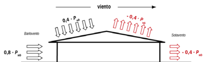
Imagen 148. Distribución de la presión eólica en un edificio con cubierta a 40° según NBE-AE88
