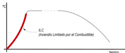
Imagen 20. Durante la fase de crecimiento, el incendio está limitado por el combustible
