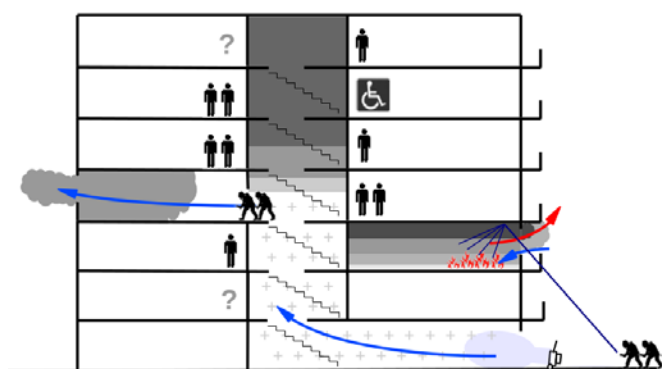
Imagen 192: Ataque exterior ofensivo "ablandado" y ataque en presión positiva para el rescate
