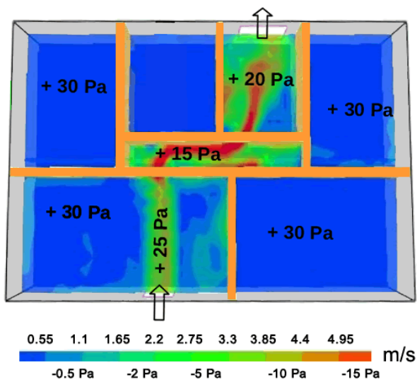
Imagen 70. Distribución de diferencias de presión y velocidades a lo largo del flujo de gases en un recinto ventilado.
