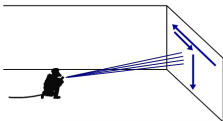
Imagen 75 : Ataque indirecto con patrón en "T".
