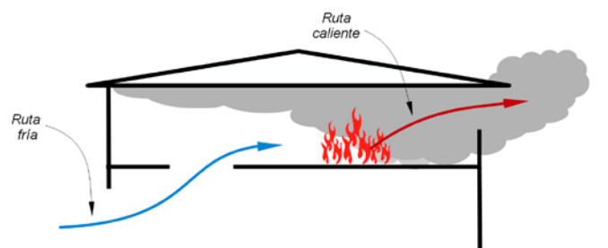
Imagen 54. Flujo de gases unidireccional generado por el incendio.
