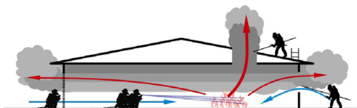
Imagen 107. Ventilación natural en cubierta.
