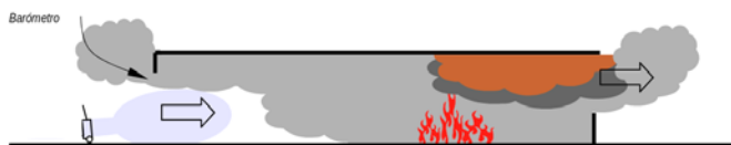
Imagen 135. Esquema general del funcionamiento del barómetro de entrada. La salida continua o creciente de gases a través del hueco deliberadamente dispuesto en la parte superior indica que la ventilación no funciona correctamente.
