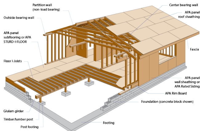
Imagen 163: Estructura de entramado ligero.
