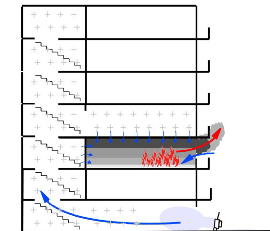
Imagen 185: Ataque en presión positiva contra la propagación
