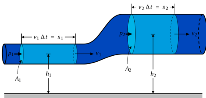
Imagen 50. Esquema de una conducción para la aplicación de la Ecuación de Bernoulli.
