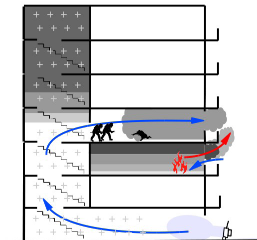
Imagen 183: Ataque en presión positiva para el rescate
