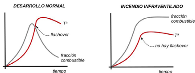
Imagen 28. Comparación de la fracción de combustible y temperatura en un incendio de desarrollo normal y en un incendio infraventilado.
