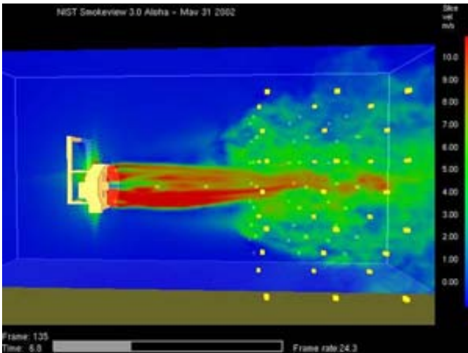
Imagen 129. Huella de un ventilador VPP en FDS (Fire Dynamic Simulator). Se aprecia el dardo de alta velocidad y el bulbo de aire succionado.
